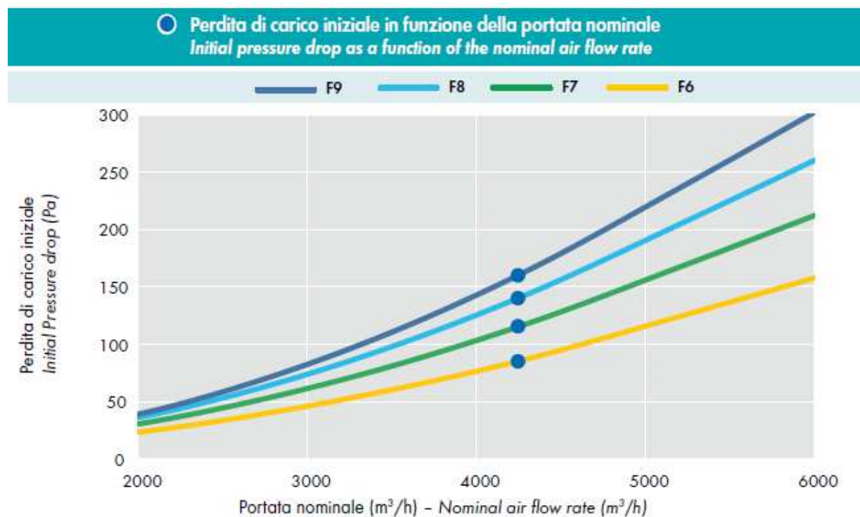
Diagramma delle perdite di carico per tasca dimensioni 592x592x292
